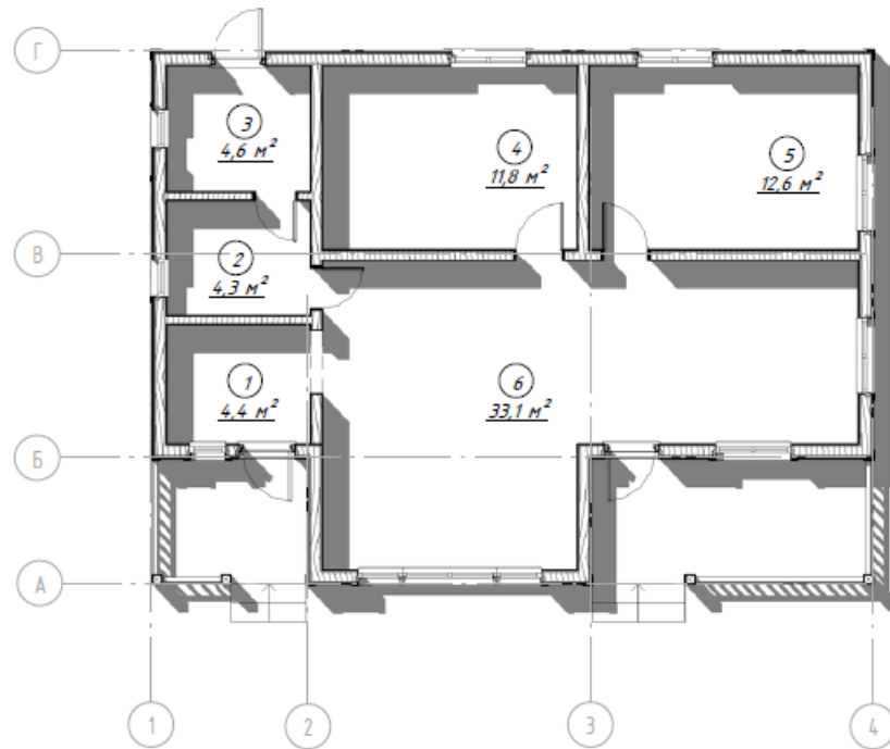
План помещений 1-го этажа
